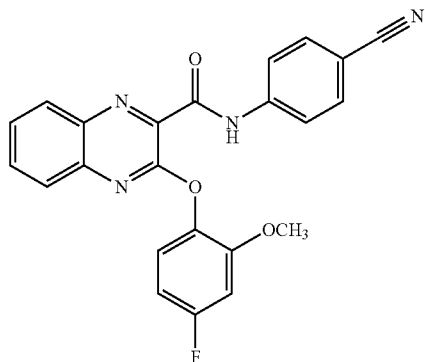
N-(4-cyanophenyl)-3-(4-fluoro-2-methoxyphenoxy)quinoxaline-2-carboxamide
