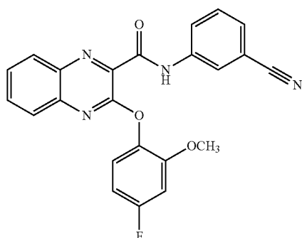
N-(3-cyanophenyl)-3-(4-fluoro-2-methoxyphenoxy)quinoxaline-2-carboxamide
