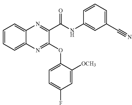
N-(3-cyanophenyl)-3-(4-fluoro-2-methoxyphenoxy)quinoxaline-2-carboxamide
