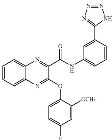
N-(3-(1H-tetrazol-5-yl)phenyl)-3-(4-fluoro-2-methoxyphenoxy)quinoxaline-2-carboxamide
