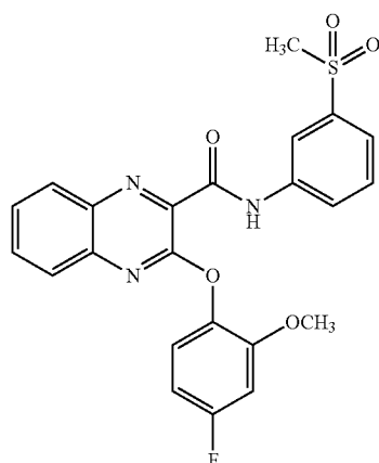
3-(4-fluoro-2-methoxyphenoxy)-N-(3-(methylsulfonyl)phenyl)quinoxaline-2-carboxamide
