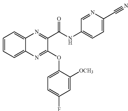
N-(6-cyanopyridin-2-yl)-3-(4-fluoro-2-methoxyphenoxy)quinoxaline-2-carboxamide
