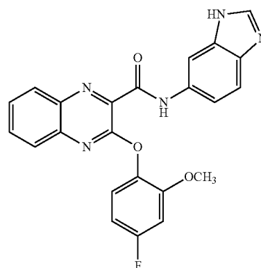
N-(1H-benzo[d]imidazol-6-yl)-3-(4-fluoro-2-methoxyphenoxy)quinoxaline-2-carboxamide
