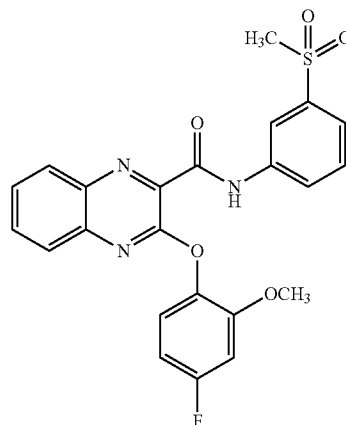
3-(4-fluoro-2-methoxyphenoxy)-N-(3-(methylsulfonyl)phenyl)quinoxaline-2-carboxamide
