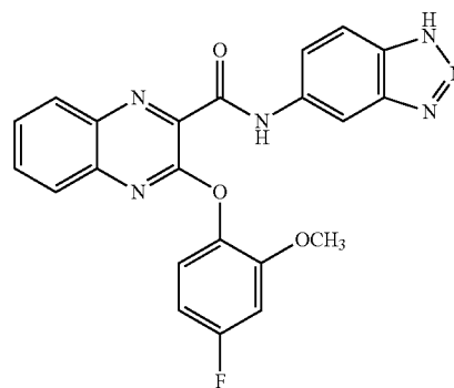
N-(1H-benzo[d][1,2,3]triazol-5-yl)-3-(4-fluoro-2-methoxyphenoxy)quinoxaline-2-carboxamide
