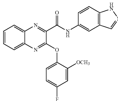
3-(4-fluoro-2-methoxyphenoxy)-N-(1H-indazol-5-yl)quinoxaline-2-carboxamide
