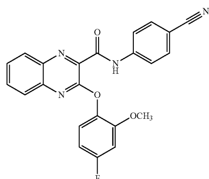
N-(4-cyanophenyl)-3-(4-fluoro-2-methoxyphenoxy)quinoxaline-2-carboxamide
