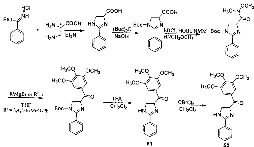
Scheme 8A
