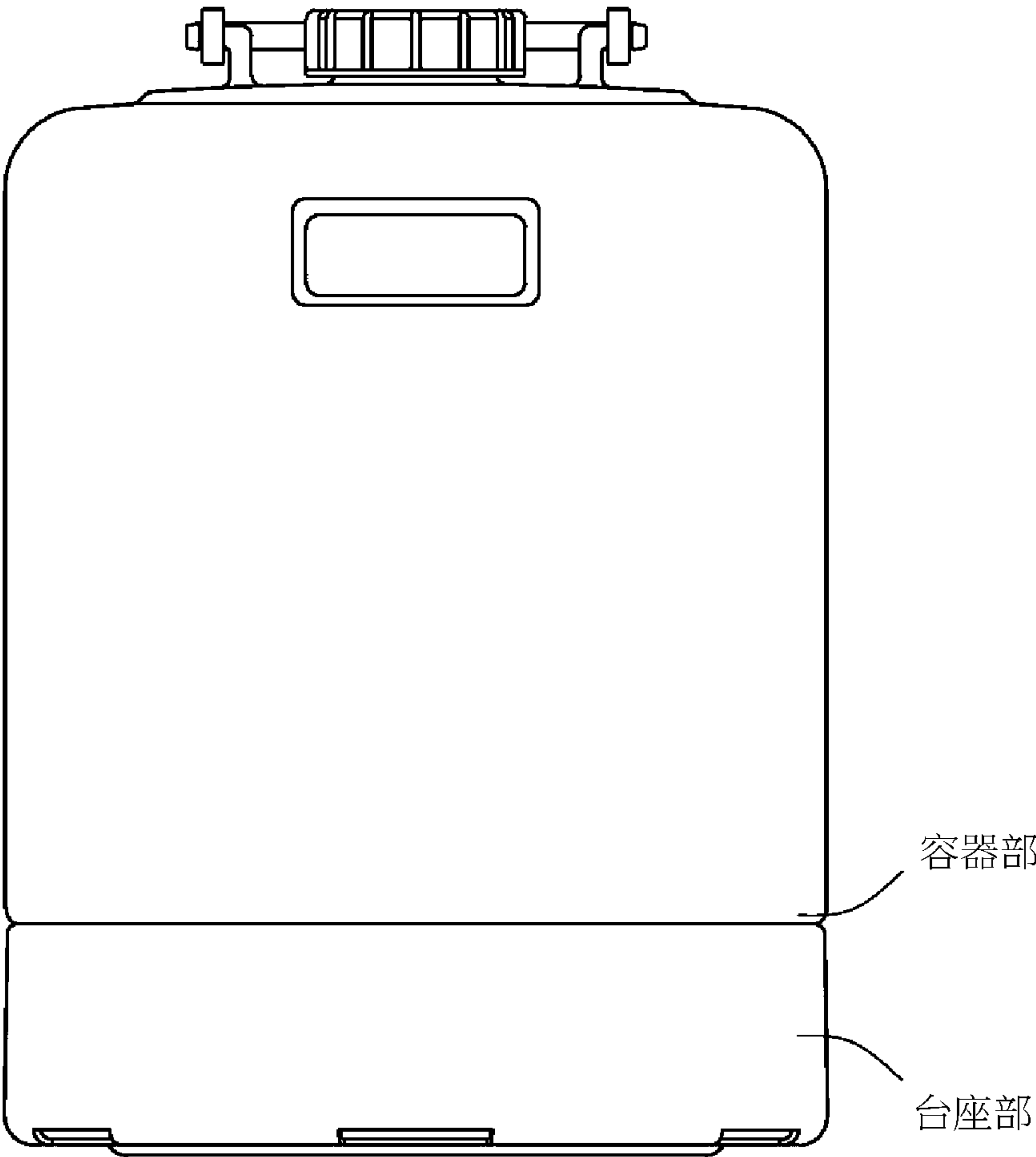
【表示使用狀態之前視參考圖】
