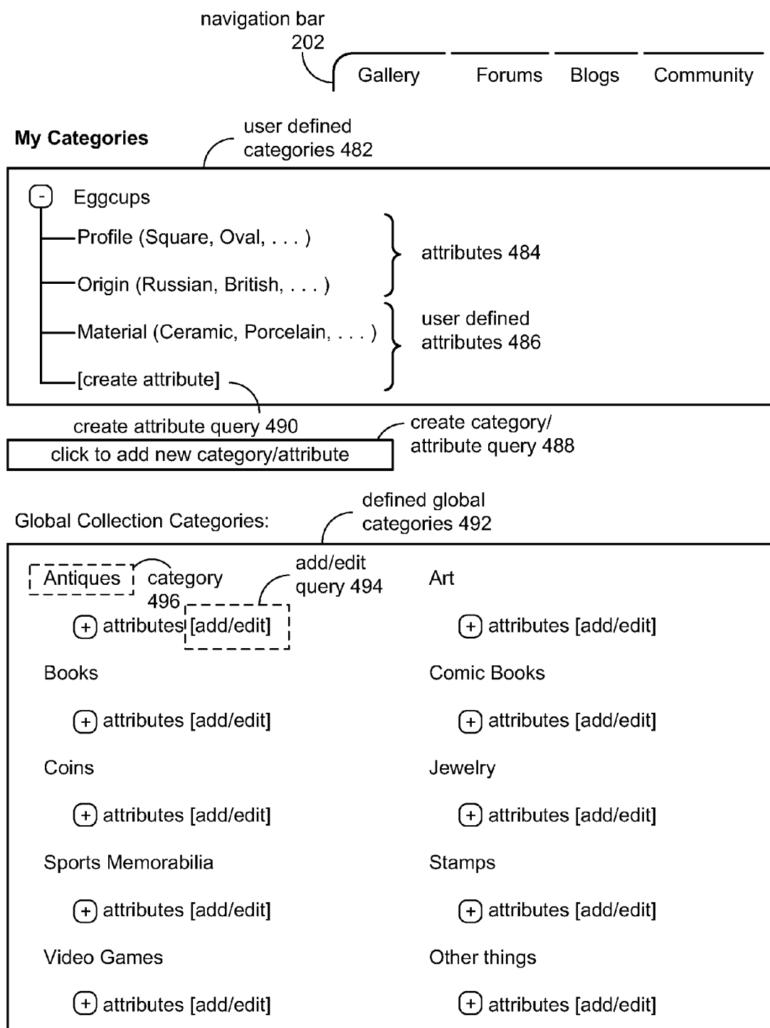
FIG. 15 category GUI 480
