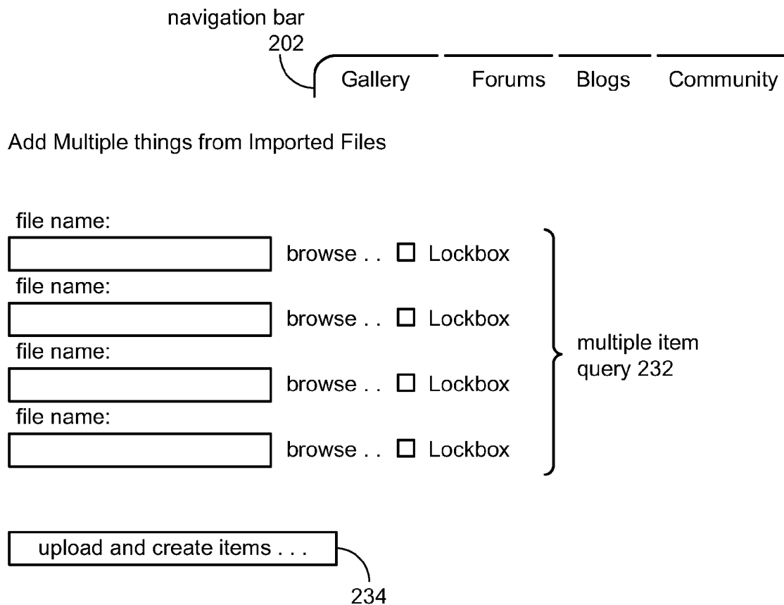
FIG. 6 rapid item import GUI 230
