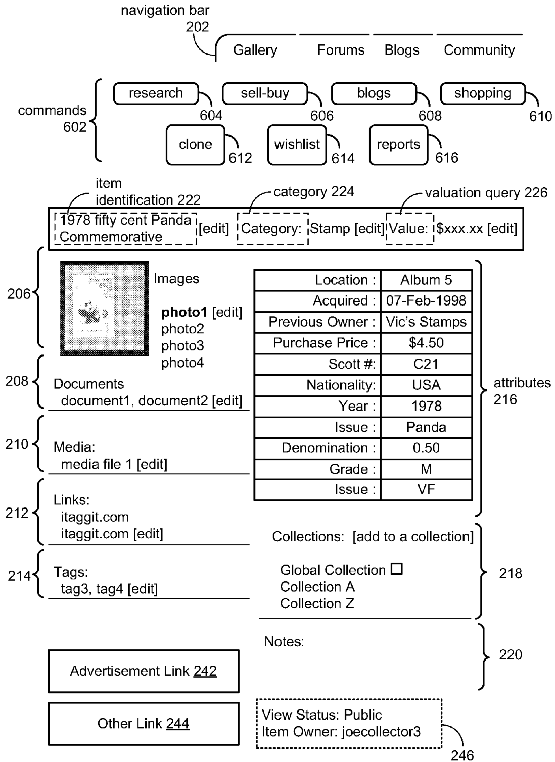
FIG. 21 web page 600
