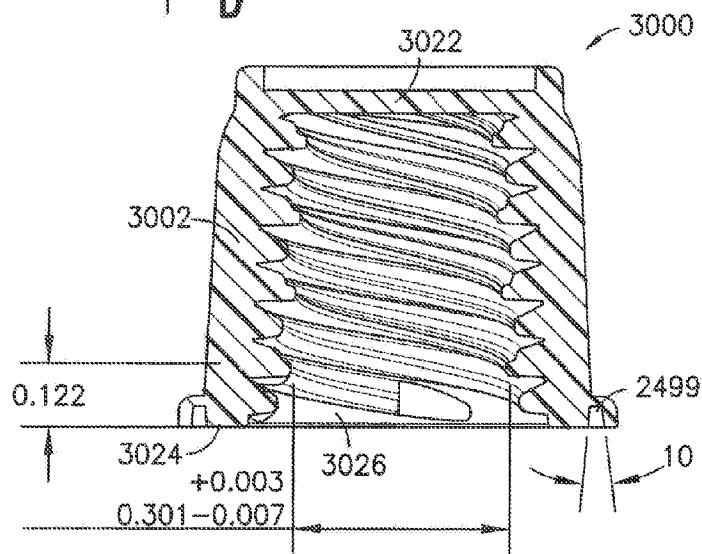
SECTION AC-AC FIG. 24E
