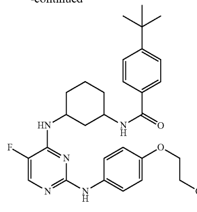
Example 1. 4-(tert-butyl)-N-(3-((5-fluoro-2-((4-(2-methoxyethoxy)phenyl)amino)pyrimidin-4-yl)amino)cyclohexyl)benzamide (3)
