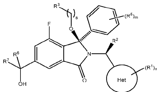
Diastereoisomer 1A
