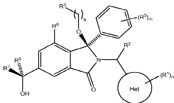
Diastereoisomer 2A
