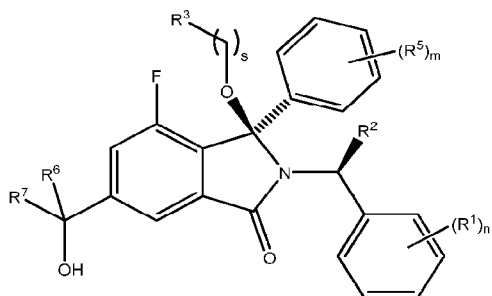
Diastereoisomer 1A
