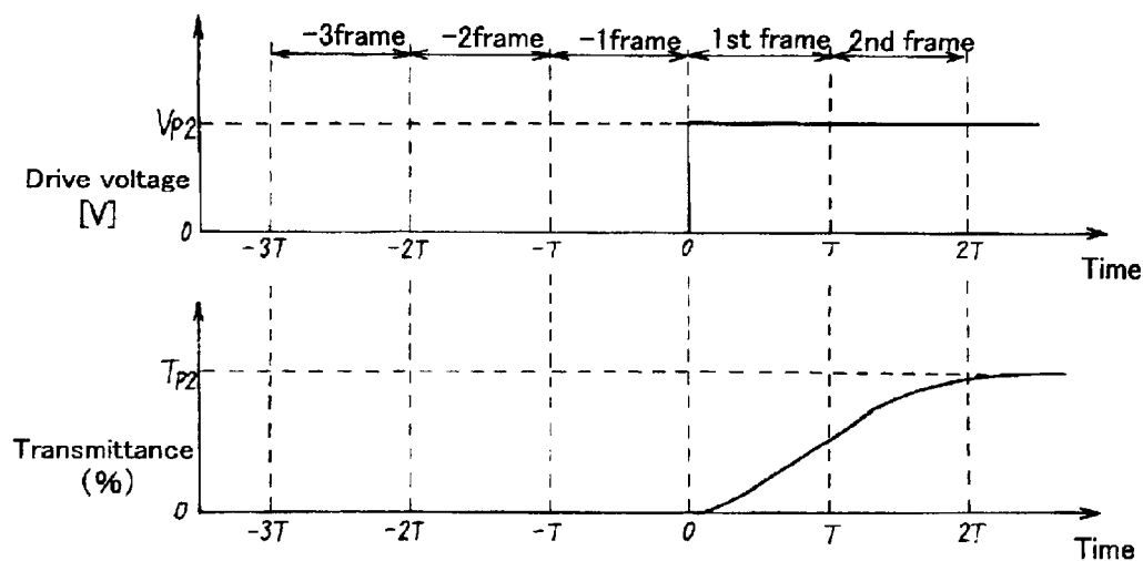
FIG. 20A No Compensation
