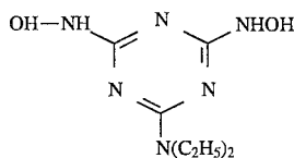
Compound (d)
