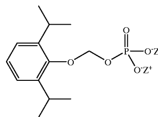
Propofol Prodrug
