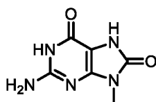
8-oxoguanine
