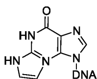
N 2 ,3-etheno-guanine
