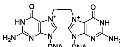
1,2-bis-(7-guanyl)-ethane
