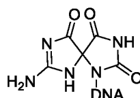
spiroiminodihydantoin Sp
