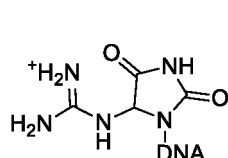
guanidinohydantoin Gh
