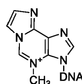
1,N 6 -etheno- adenine
