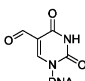
5-formyluracil
