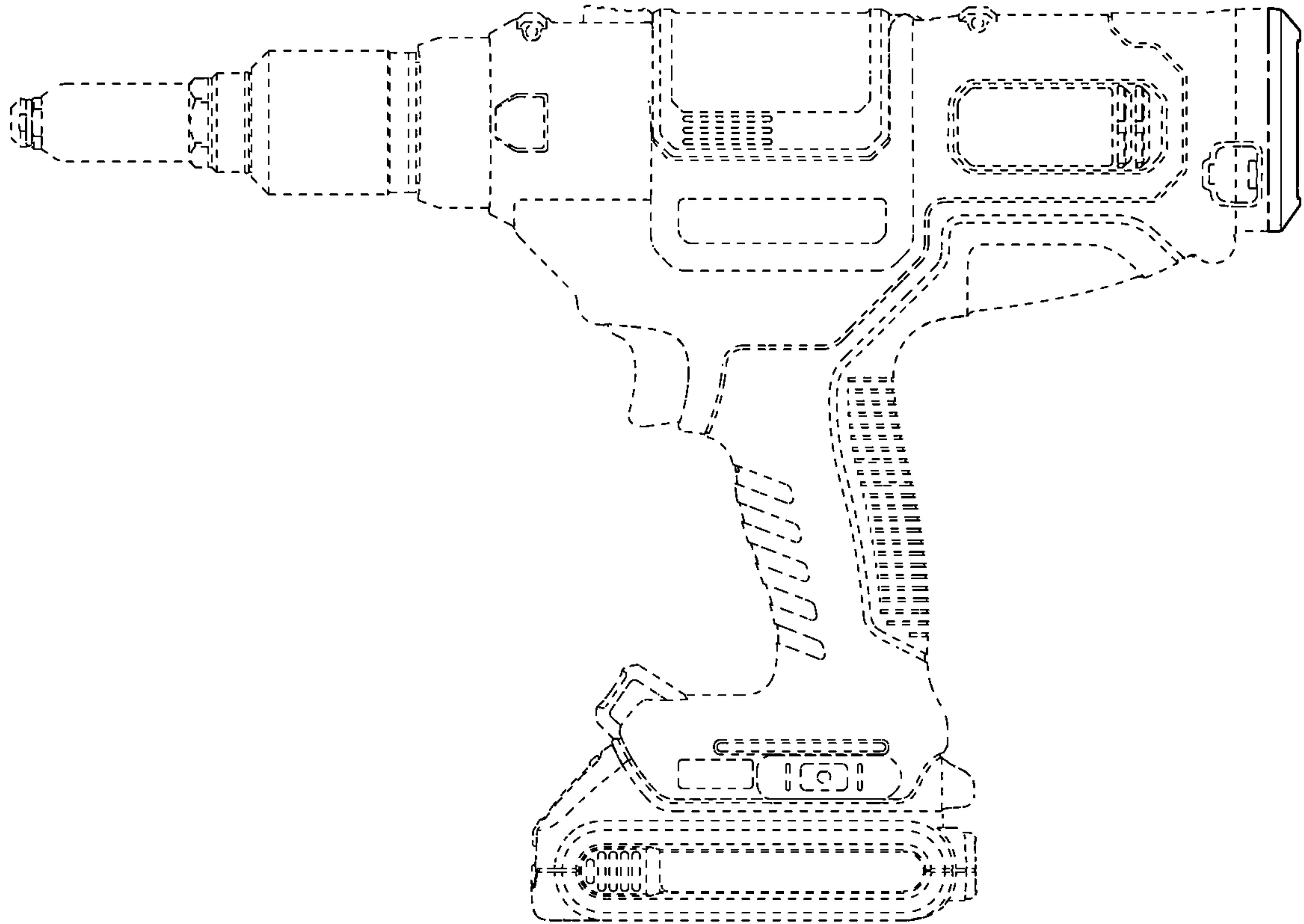
【前視圖】
