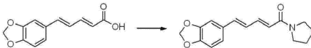
(2E,4E)-5-(benzo[d][1,3]dioxol-5-yl)-1-(pyrrolidin-1-yl)penta-2,4-diene-1-one (LJ-2487)
