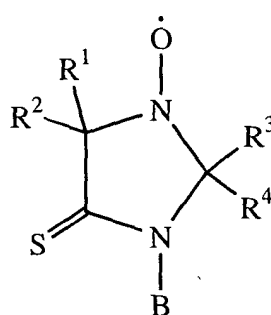
(Vb)
