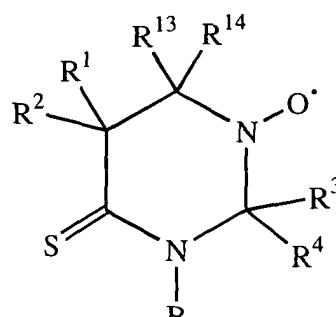
(VIIb)
