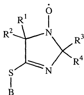
(Va)
