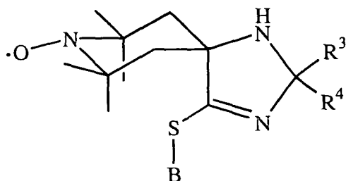
(VIa)
