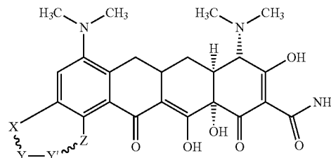
Formula A1
