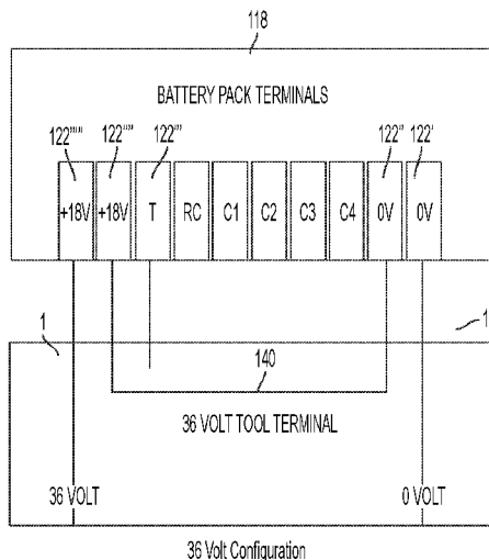
36 Volt Configuration
