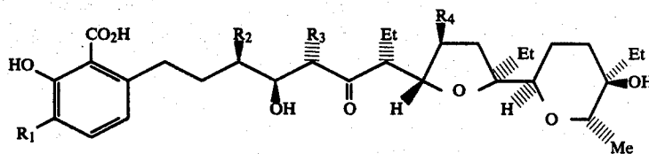
Iso-Lasalocid A
