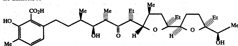
Iso-Lasalocid A
