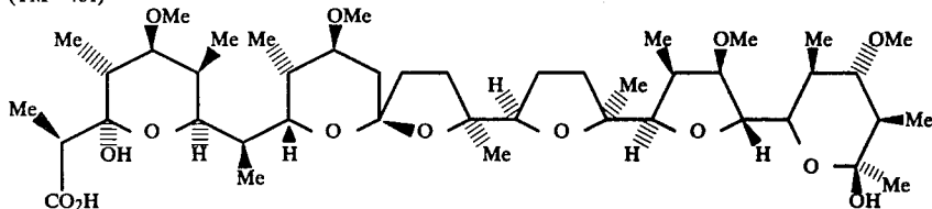
Lonomycin (TM - 481)
