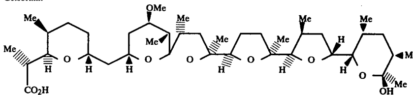
Grisorixin
