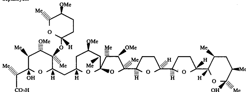
Septamycin
