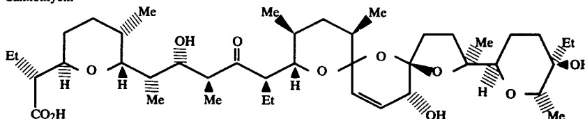
Salinomycin
