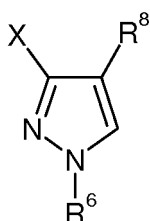
1,3-isomer
