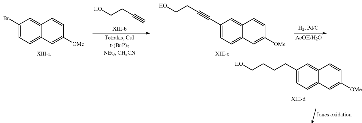
Scheme XIII 3,5-diamino-N-(N-(4-(6-((S)-4-amino-3-(3-(bis((2S,3R,4R,5R)-2,3,4,5,6-pentahydroxyhexyl)amino)propylamino)-4-oxobutyl)naphthalen-2-yl)butyl)carbamimidoyl)-6-chloropyrazine-2-carboxamide
