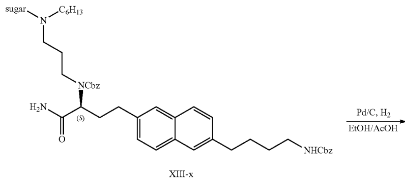
Scheme XIV 3,5-diamino-N-(N-(4-(6-((S)-4-amino-3-(3-hexyl((2S,3R,4R,5R)-2,3,4,5,6-pentahydroxyhexyl)amino)propylamino)-4-oxobutyl)naphthalen-2-yl)butyl)carbamidoyl)-6-chloropyrazine-2-carboxamide
