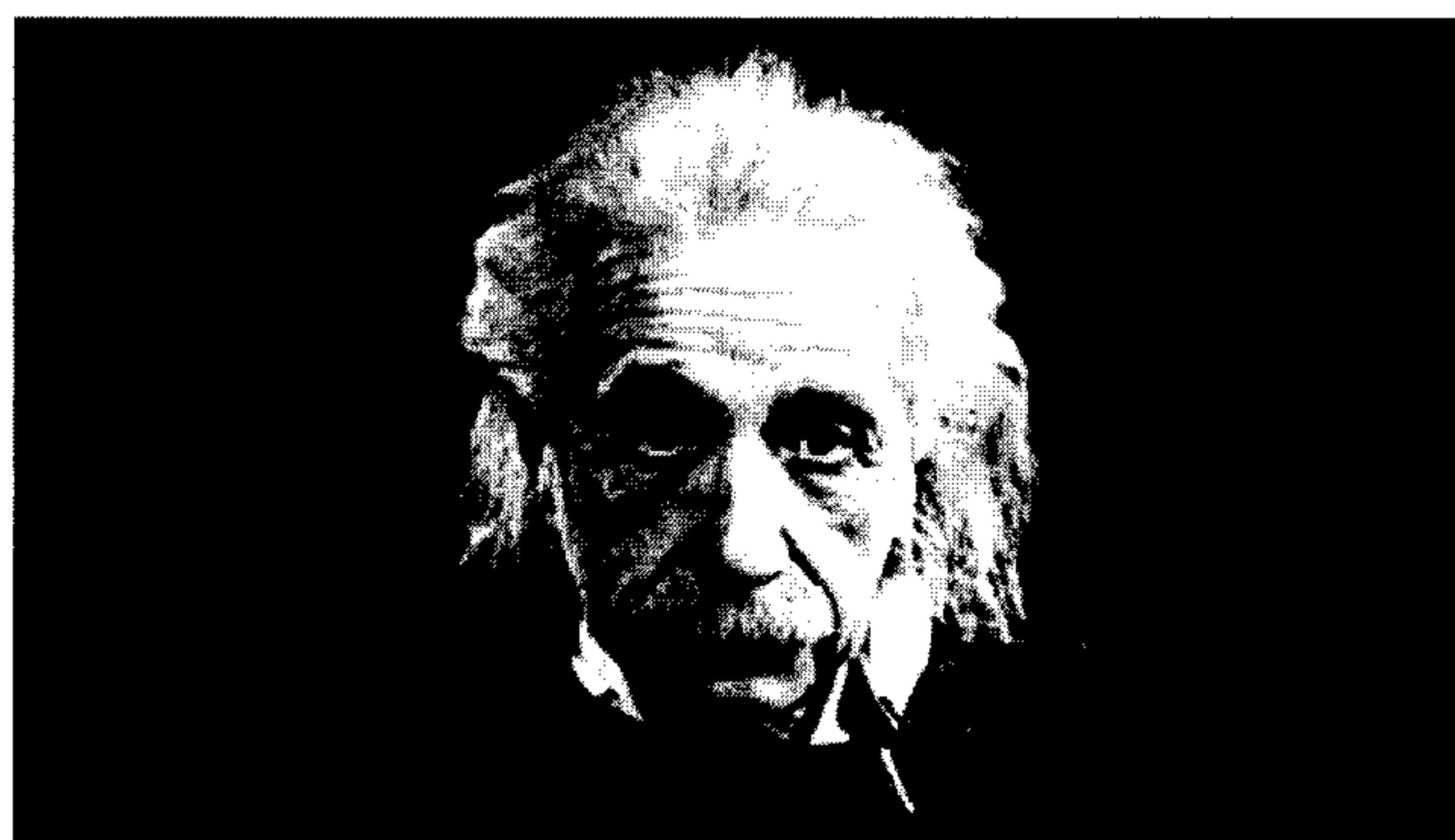
FIG. 28E target
