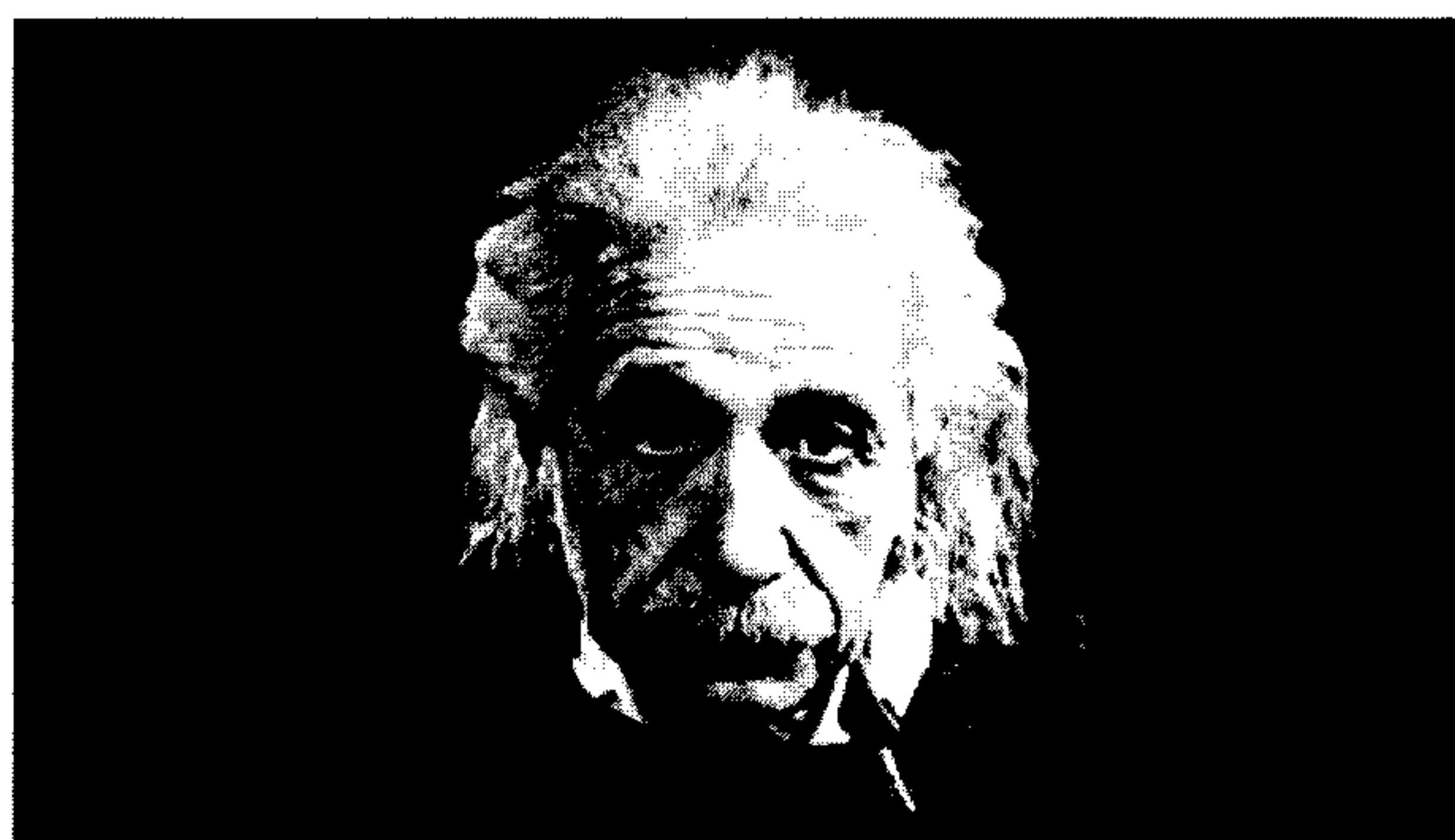
FIG. 26E target
