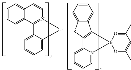
Ir(piq) 3
