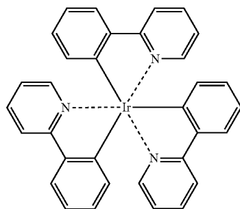
Ir(ppy) 3
