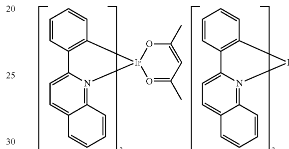
Ir(pq) 2 (acac)
