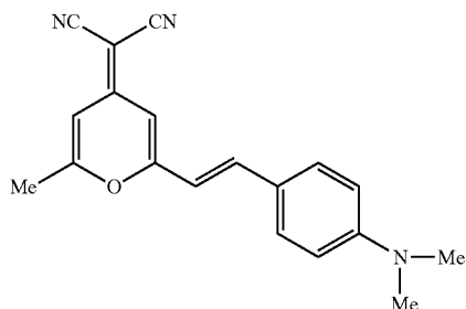
DCM
