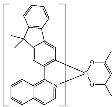
Ir(fliq) 2 (acac)
