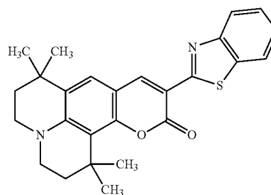
C545T
