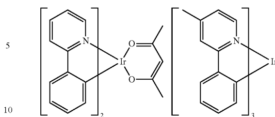
Ir(ppy) 2 (acac)
