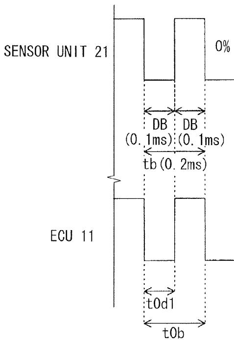
FIG. 13B SG : 0% DUTY
