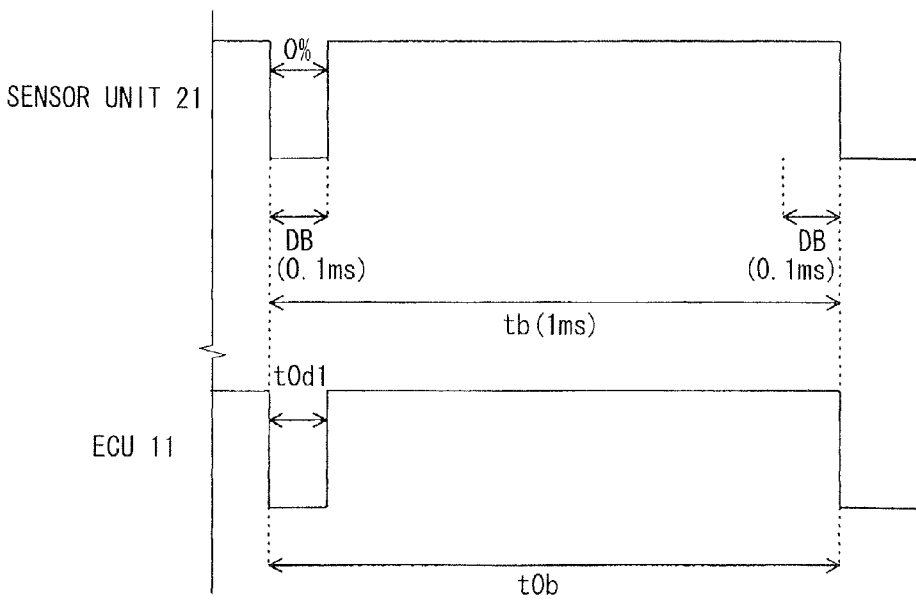
FIG. 3B SG : 0% DUTY
