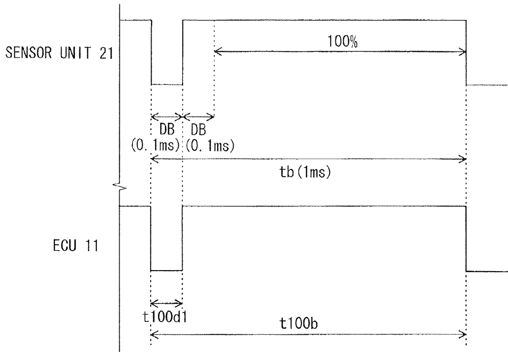
FIG. 13A SG : 100% DUTY
