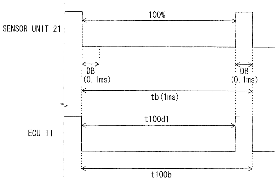
FIG. 3A SG : 100% DUTY
