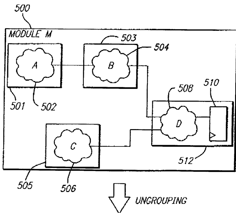
FIG. 22 HIERARCHY UNGROUPING
