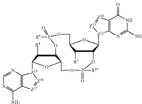
Formula Ic
