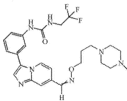
Vegyület 1-56
