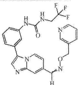
Vegyület 1-55
