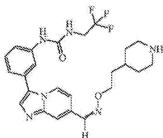
Vegyület 1-59
