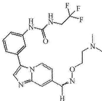
Vegyület 1-57
