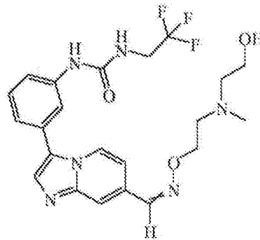
Vegyület 1-58
