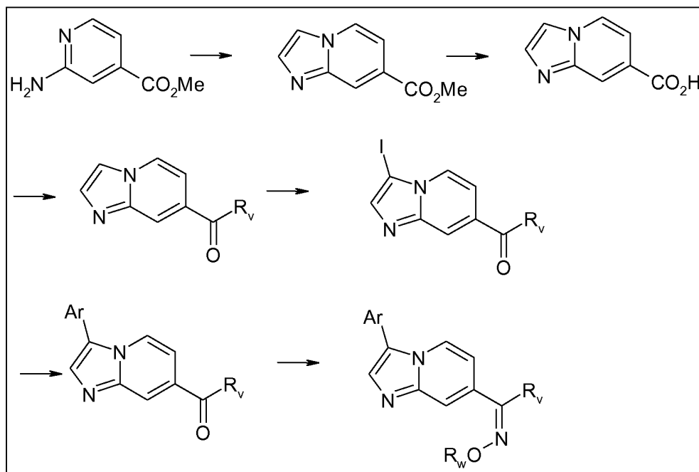
Scheme 1A
