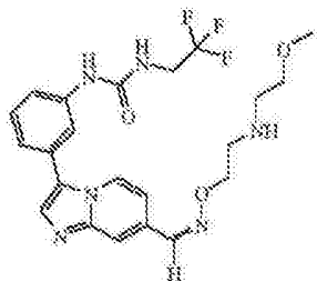
Vegyület 1-53
