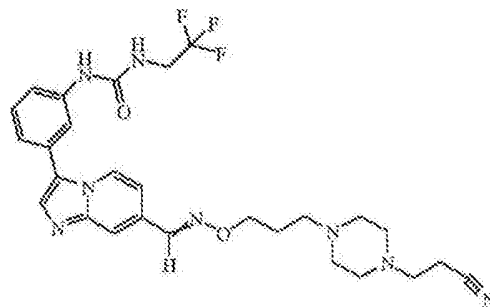
Vegyület 1-60
