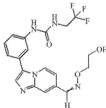
Vegyület 1-54
