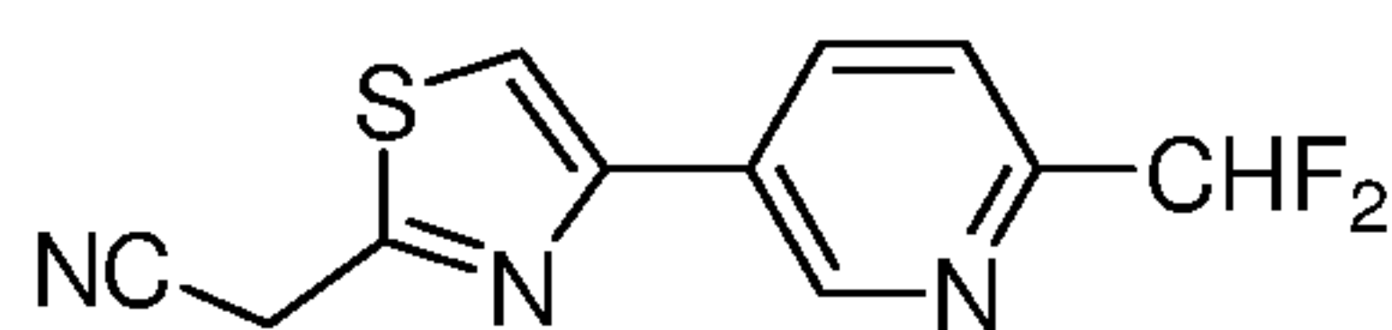
Nitrile 25
