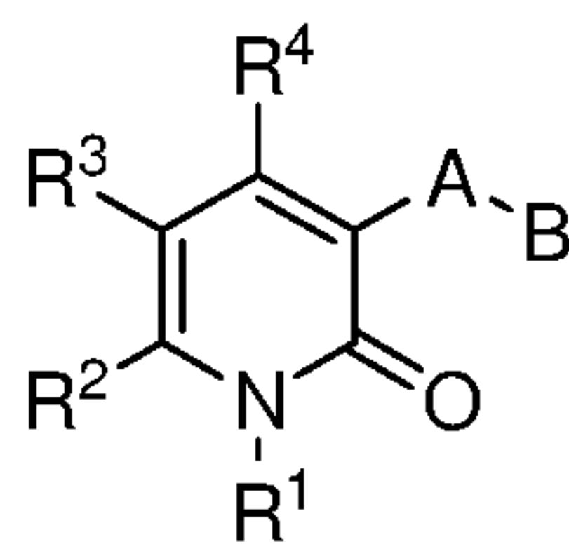
Formula (IA).
