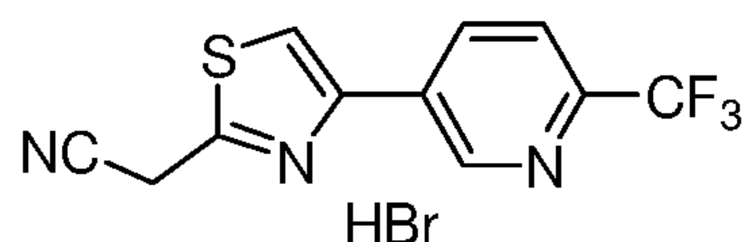
Nitrile 26
