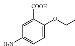
2-ethoxy-5-aminobenzoic acid
