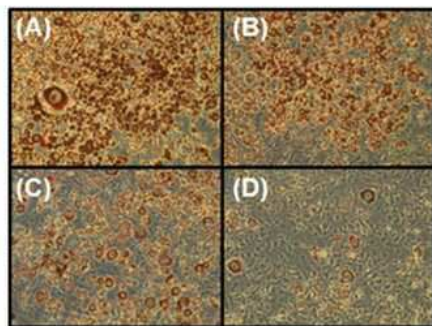
Isoalantolactone
