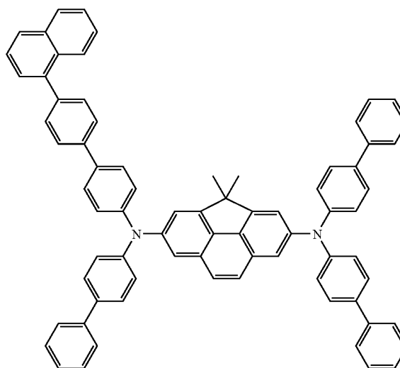
<Formula 33>
