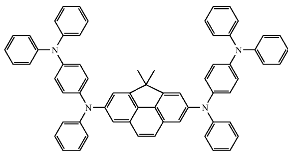
<Formula 34>
