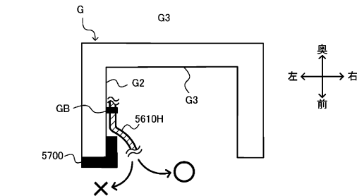
(A) ケーブルと枠部材との関係
