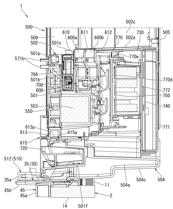
ア－ア線断面
