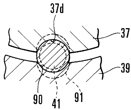
FIG. 24C
