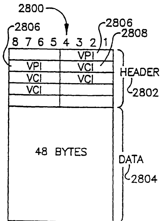
ATM CELL Fig. 28
