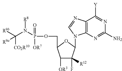
Formula Ic
