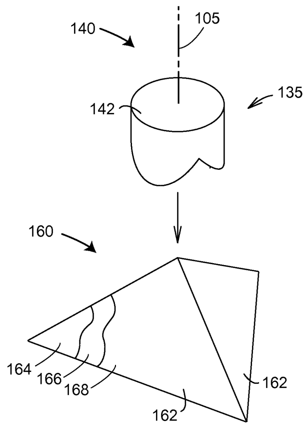
FIG. 1E PRIOR ART
