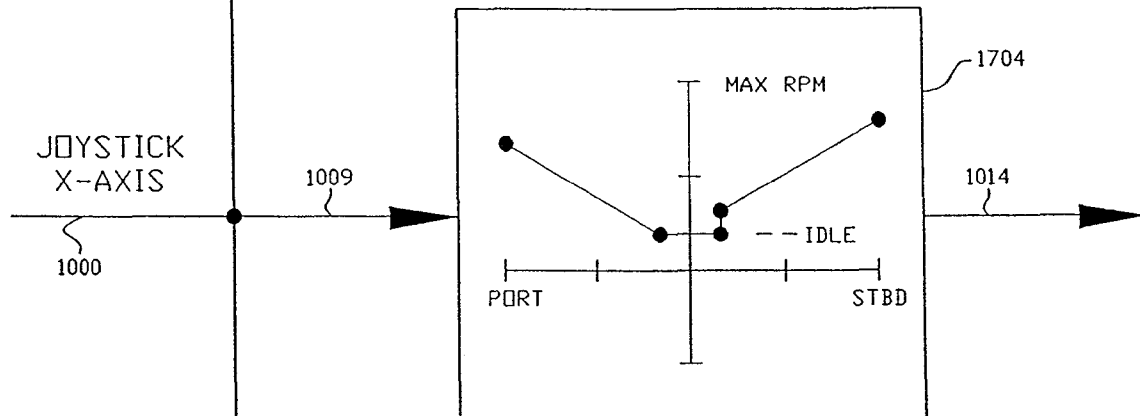
FIG. 15E STBD ENGINE RPM
