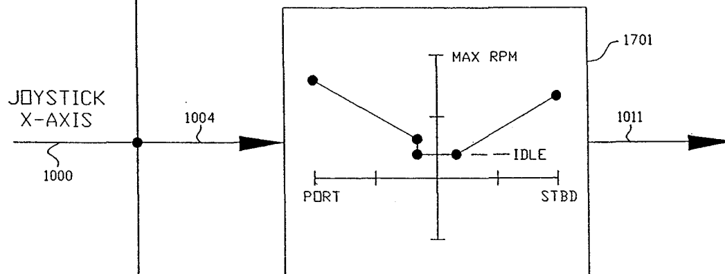
FIG. 14E PORT ENGINE RPM
