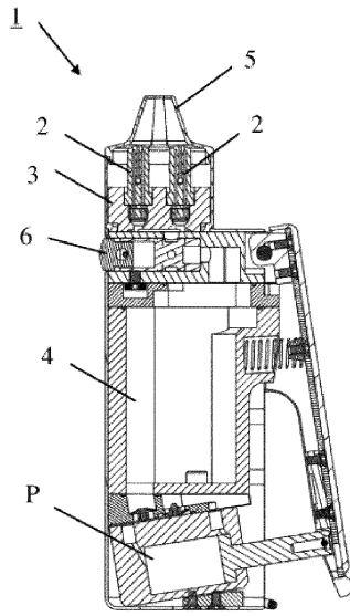
Фиг. 13
