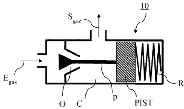
Фиг. 8
