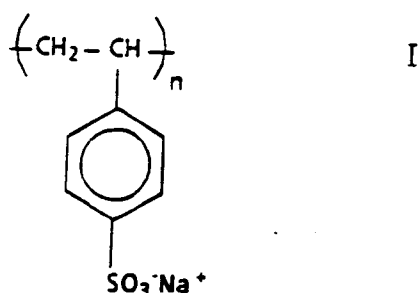
poly(sodium styrene sulfonate)
