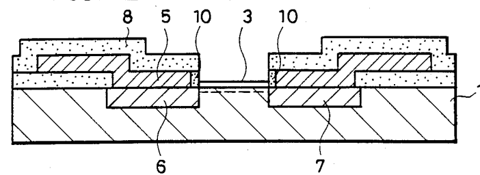
FIG. 4E PRIOR ART
