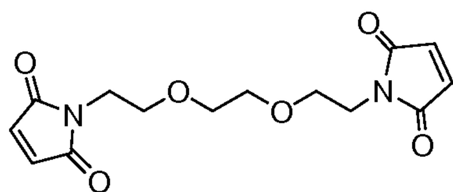
BM(PEO) 2
