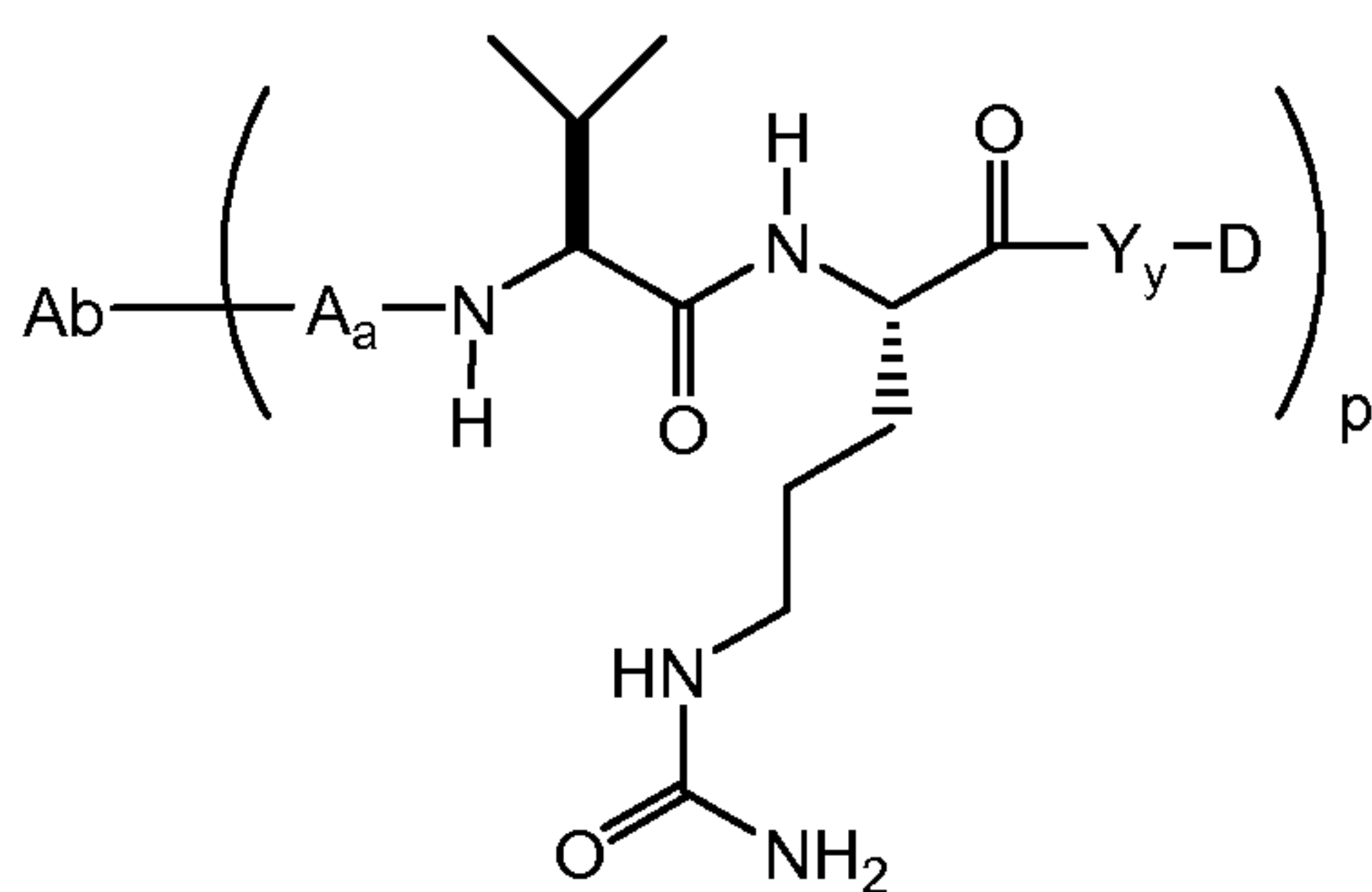
valine-citrulline (val-cit or vc)
