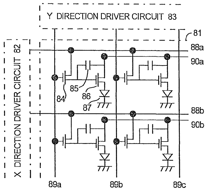
FIG. 24A EL PANEL CIRCUIT DIAGRAM
