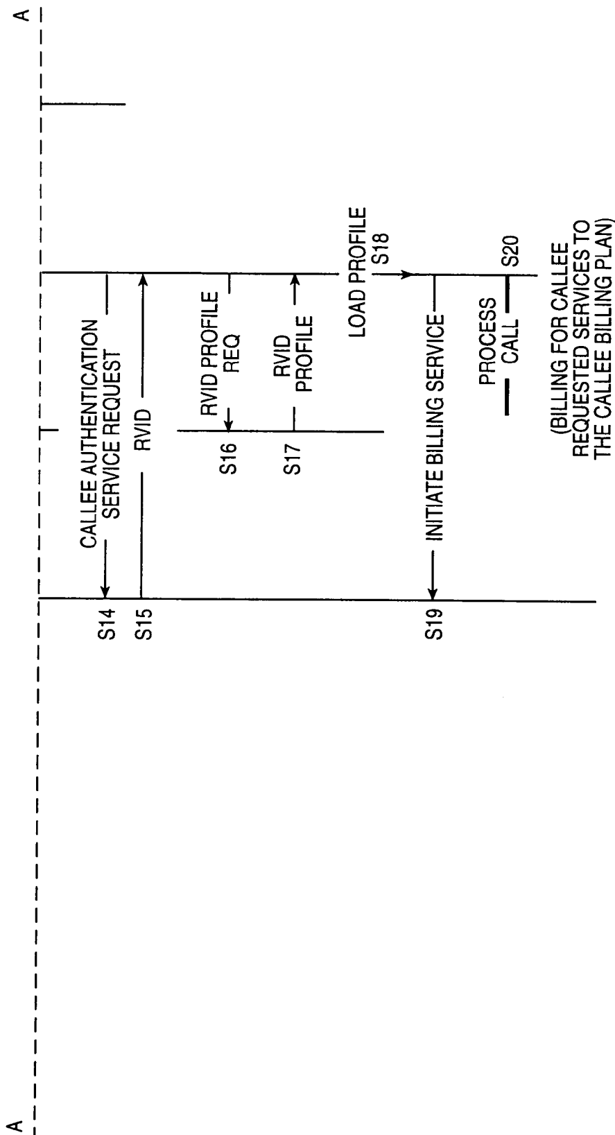
FIG. 5B
