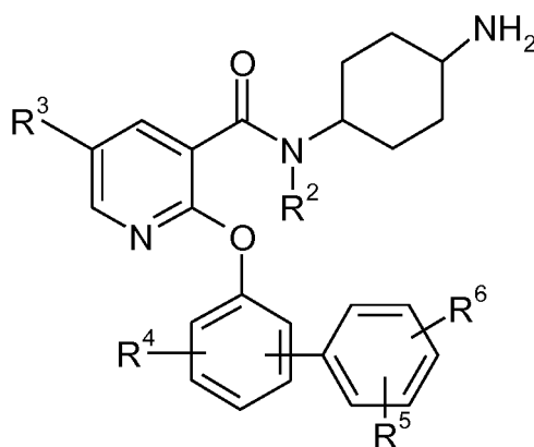
(III)
