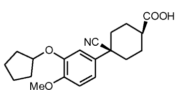
Cilomilast
