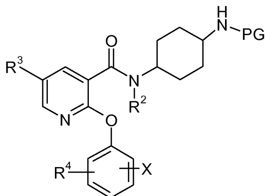
(XVII)
