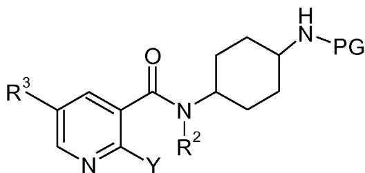
(XVI)
