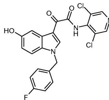
AWD 12-281
