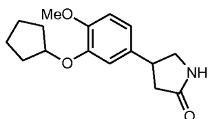
Rolipram
