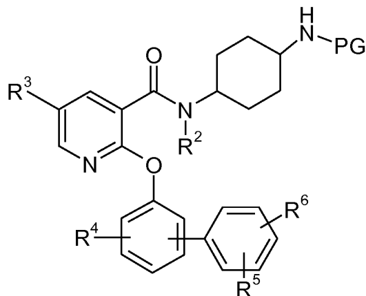
(XV)
