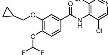
Roflumilast
