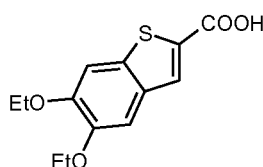
Tibtenelast
