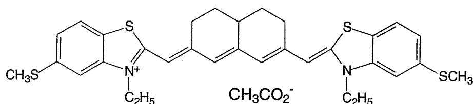
IR Dye 16
