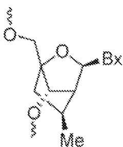
S-Me cLNA
