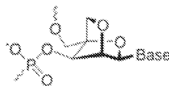
beta-D-amino-LNA
