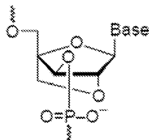
beta-D-amino-LNA
