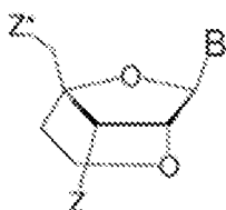
ENA
