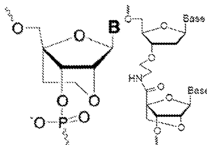
amide-linked LNA
