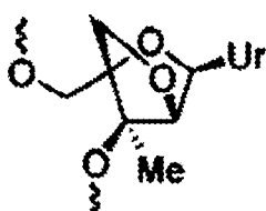
3'-Me-alpha-L-LNA
