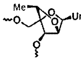
3'-Me-alpha-L-LNA
