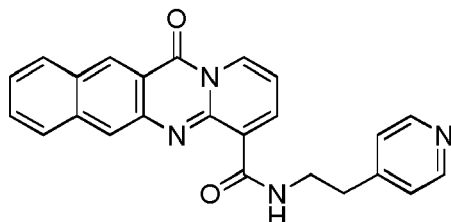
compound 37 (LI-246).
