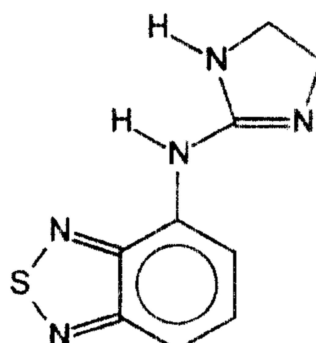
Indanazoline
