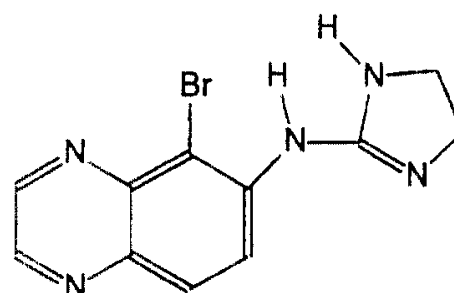
Brimonidine
