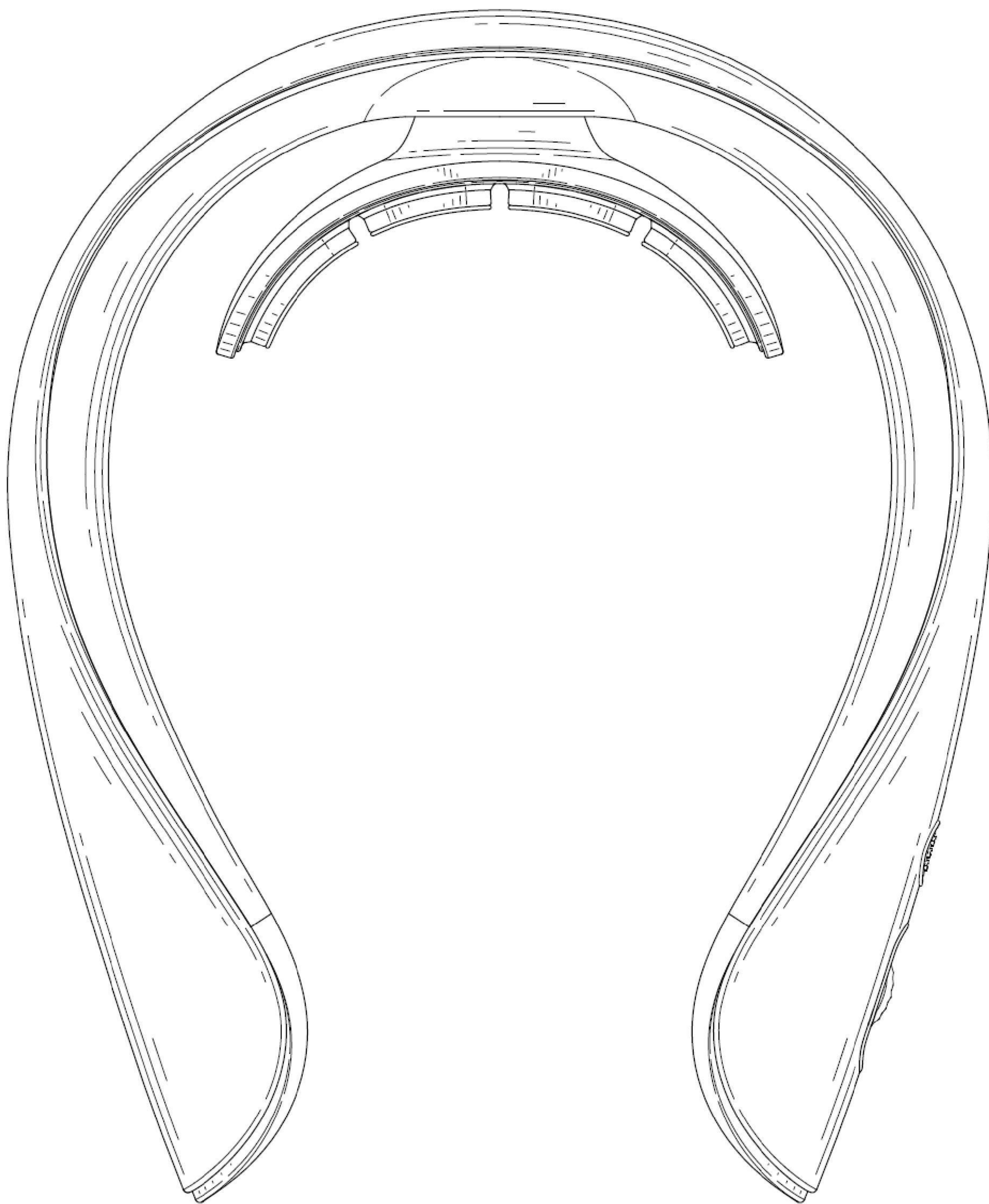
【前視圖】
