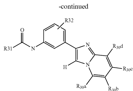
III-1a
