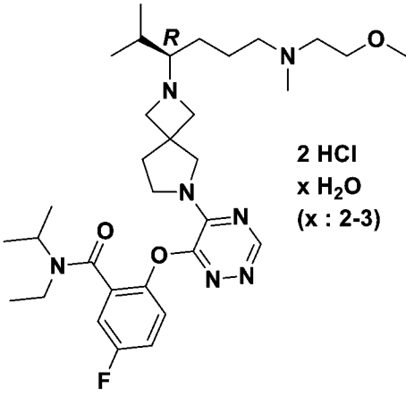
化合物A1。
