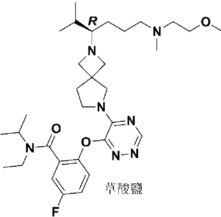
化合物A3。
