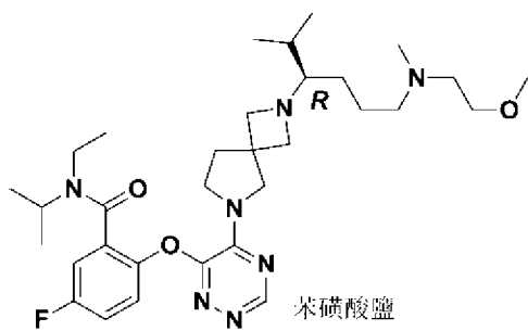
化合物A4-a
