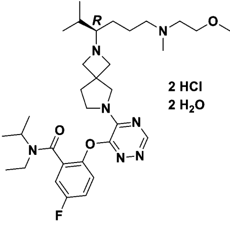
化合物A2。
